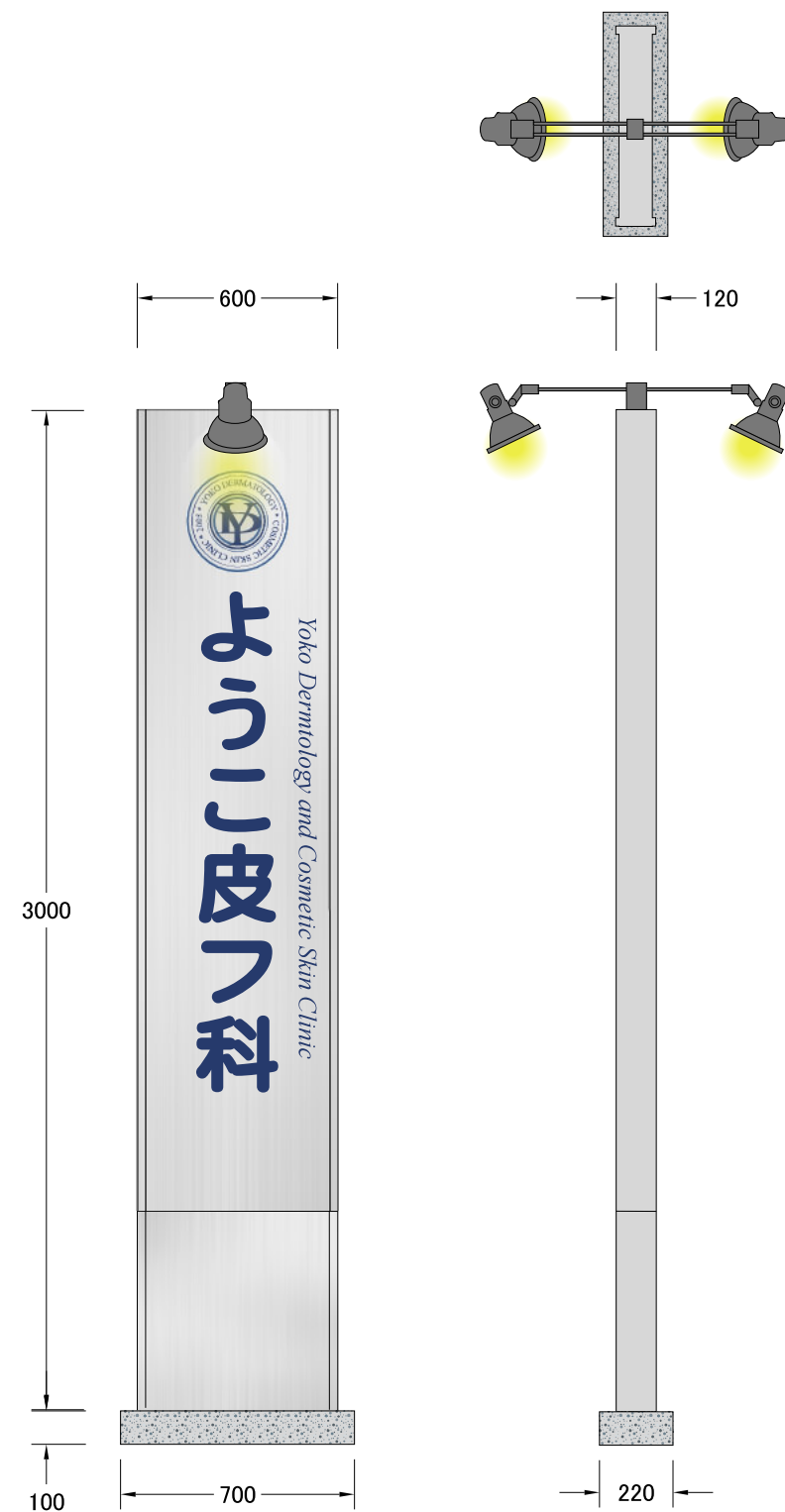
寸法図
